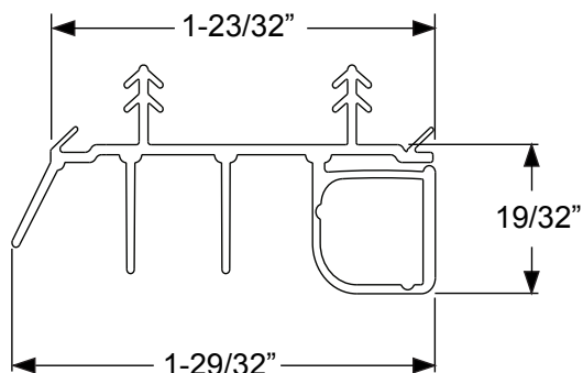
Single Bulb Kerf-Applied Door Bottom
