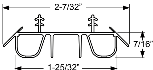
Dual Bulb Kerf-Applied Door Bottom
