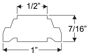
Muntin Bar
